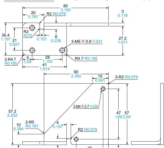
MS-LX-2 Anclaje de montaje del sensor (Opcional)
